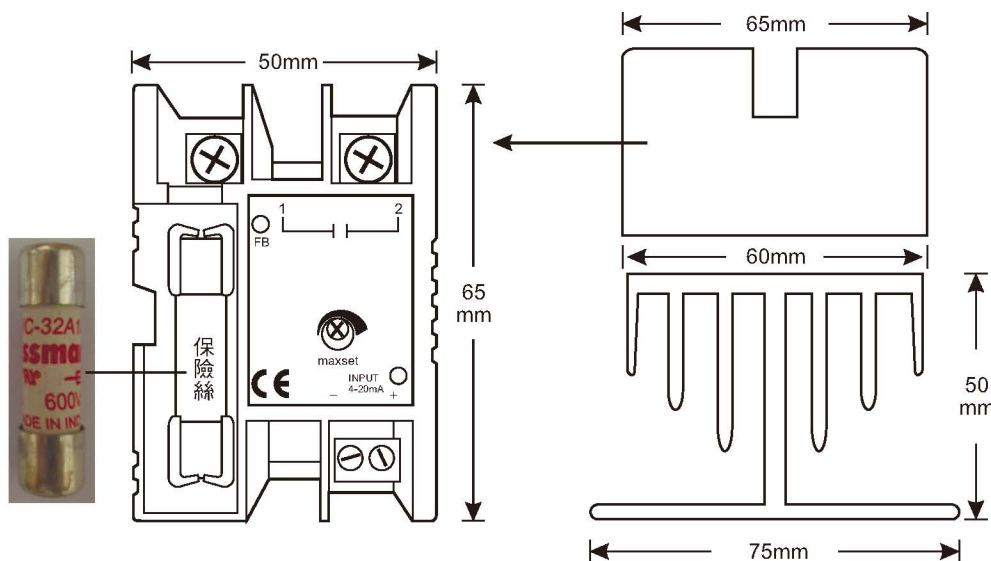
散熱片尺寸
